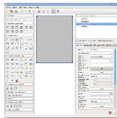
Glade / Gazpacho
