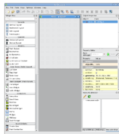
QtDesigner
